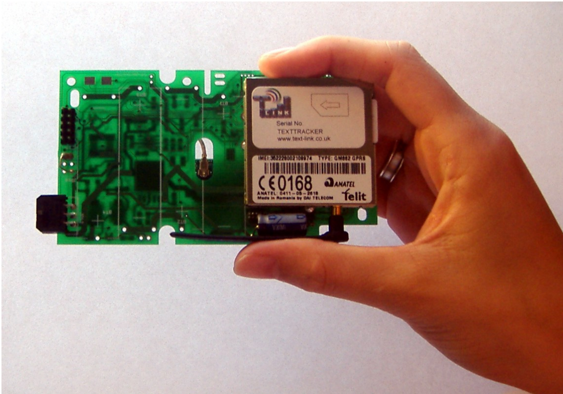
Textlink Ltd - GSM Interface Module: 117mm x 69mm
